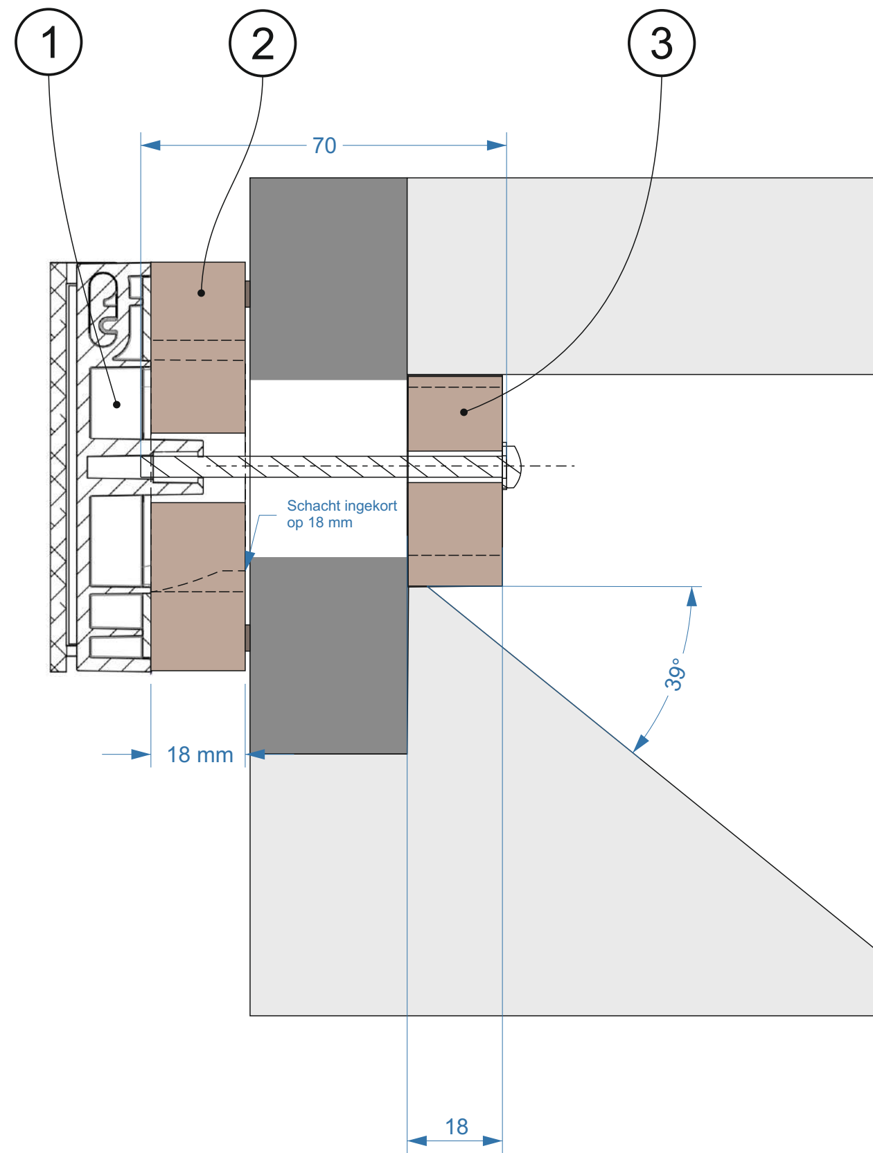
Doorsnede A-A
