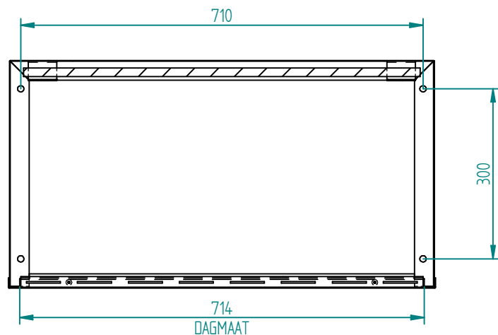
DOORSNEDE A-A
