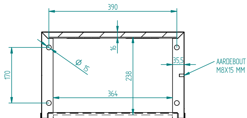
DOORSNEDE A-A
